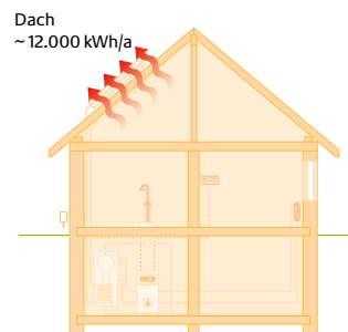
Jährliche Wärmeverluste ohne Dachdämmung
