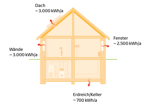
Jährliche Wärmeverluste mit Dachdämmung
