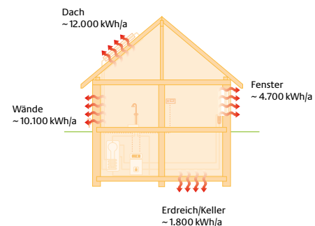
Jährliche Wärmeverluste ohne Dachdämmung
